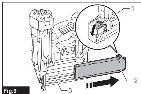
► 1. Levier 2. Porte coulissante 3. Magasin
