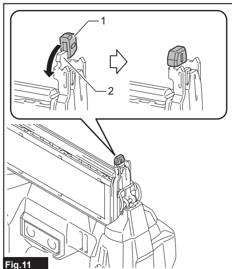
► 1. Adaptateur de bec 2. Élément de contact
