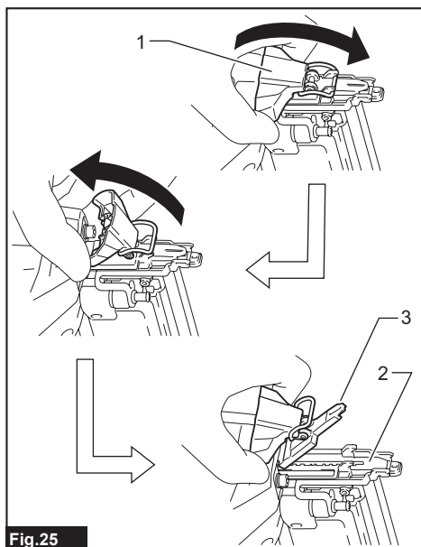
► 1. Seguro 2. Guía inferior del impulsor 3. Guía del impulsor
