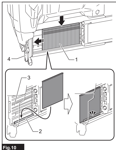
► 1. Bande de fixations 2. Plaque de magasin 3. Magasin 4. Guide d'entraînement
