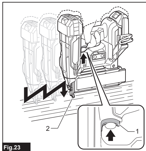
► 1. Gatillo interruptor 2. Elemento de contacto
